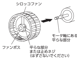
シロッコファン
